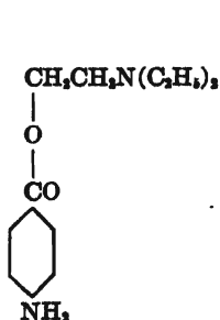
Novocaine
