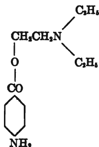
Procaine
