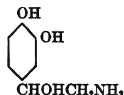
XXI
