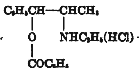
XXVI
