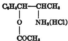
XXII
