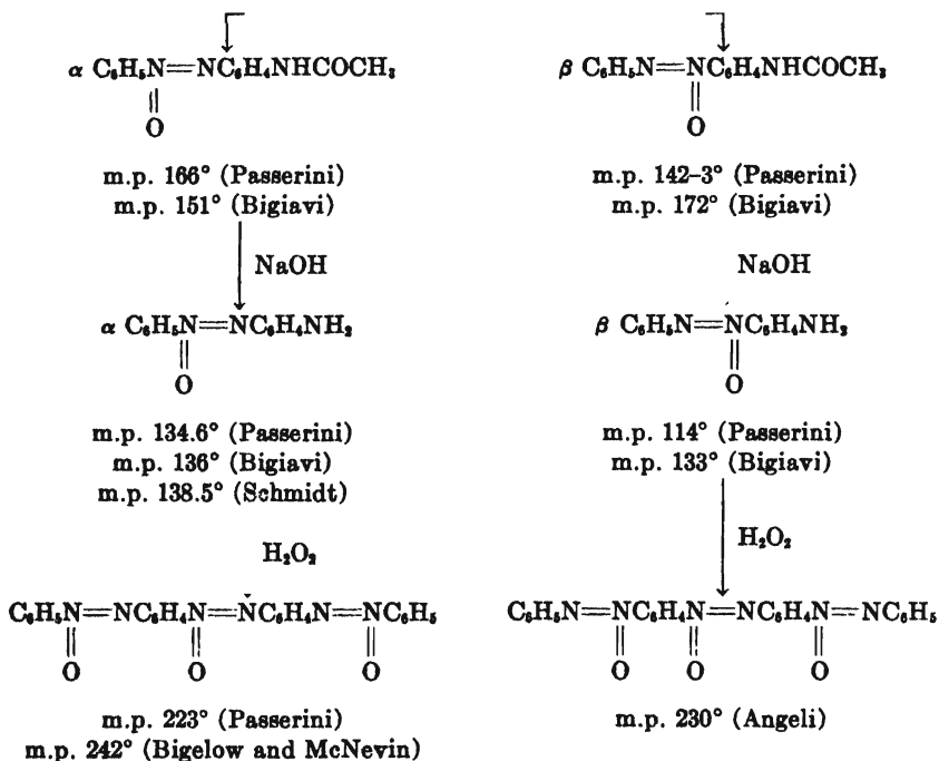
FIG. 12. SYNTHESIS OF TRISAZOXYBENZENES
