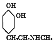
XX
