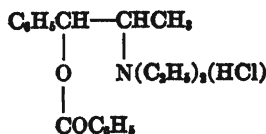
XXVII
